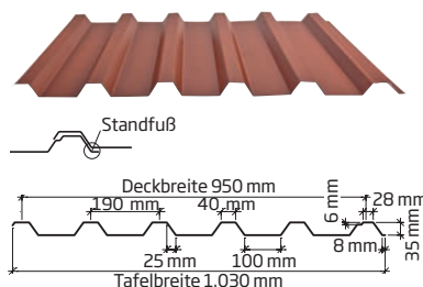
DS Trapez TP 35-190
