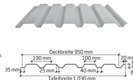
DS Trapez VP 35-190
