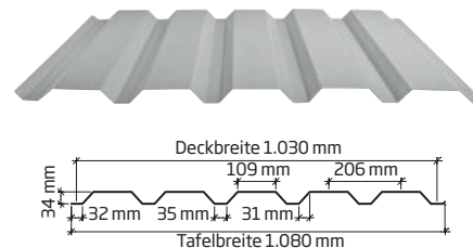
DS Trapez VP 35-206 (Mit oder ohne Designsicke)
