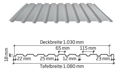
DS Trapez VP 20-115
